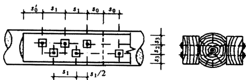
图 6.2.5-2 两纵行错列
