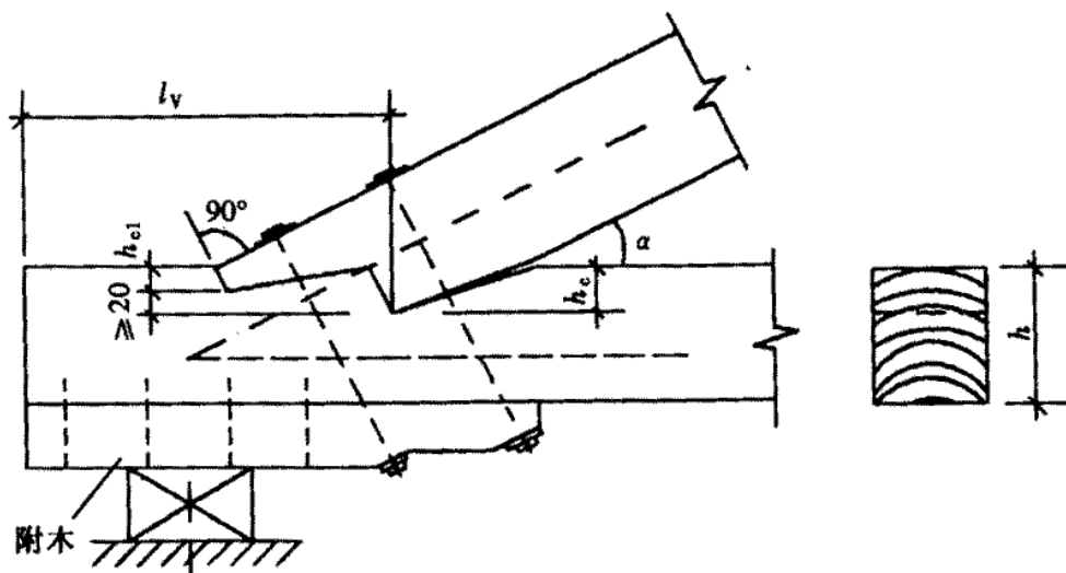
图 6.1.1-2 双齿连接
