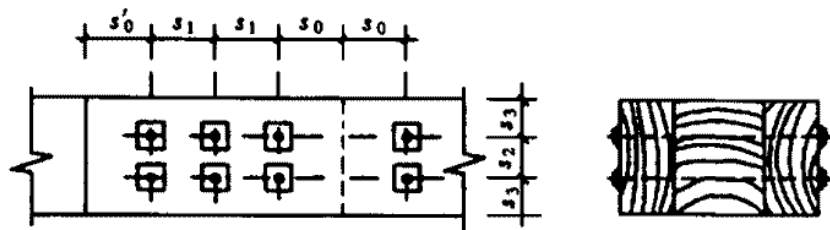
图 6.2.5-1 两纵行齐列
