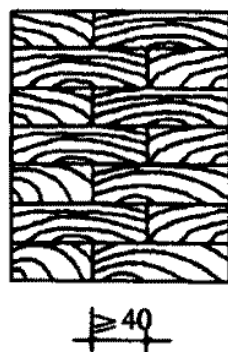
图 8.3.5 木板拼接
