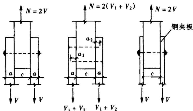
图 6.2.1-1 双剪连接
