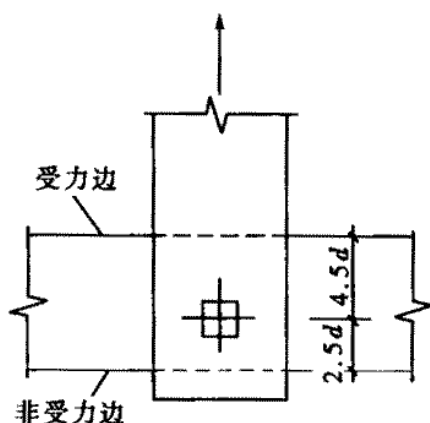
图 6.2.5-3 横纹受力时螺栓排列
