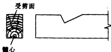
图 7.3.4 受剪面避开髓心示意图
