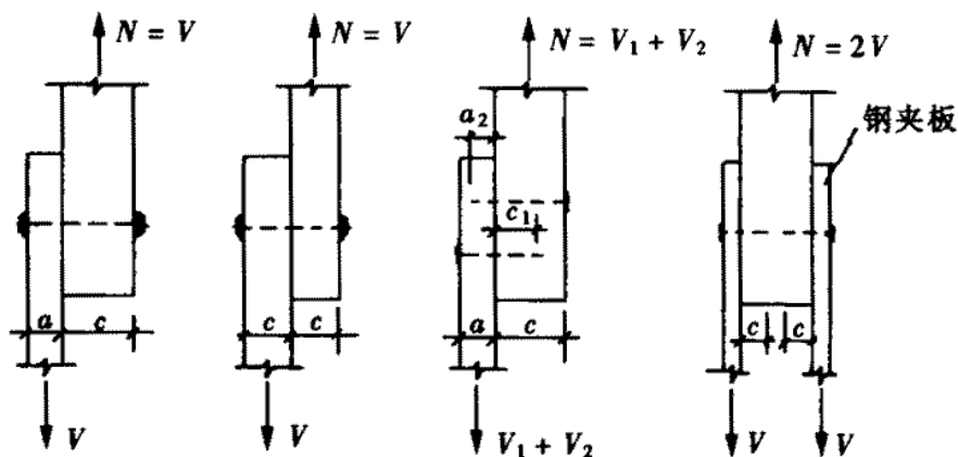
图 6.2.1-2 单剪连接
