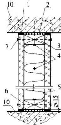
图2 分户墙及房间隔墙 竖向剖面图
