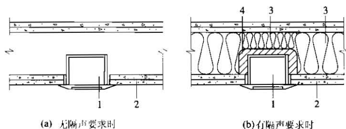
图 5.9.1 电源插座盒安装示意图
