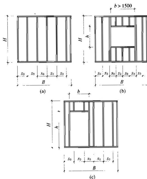
图 3.1.4 木骨架布置示意图
