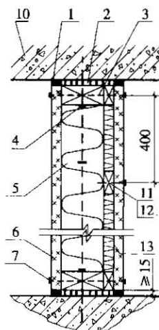
4 隔声内墙竖向剖面图
