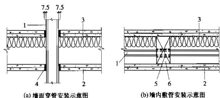
图 5.9.2 墙面穿管及墙内敷管安装示意图
