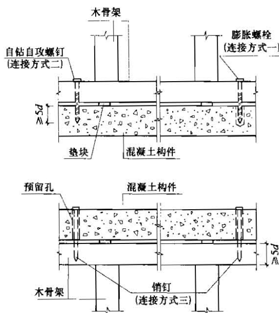
图 5.3.6 墙体与主体结构连接示意图
