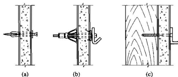
图 5.9.3 墙体上悬挂物体的固定方法示意图
