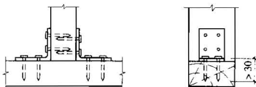
图 5.3.8 外墙木骨架构件之间角链连接示意图
