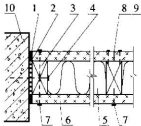
图1 分户墙及房间隔墙 水平剖面图
