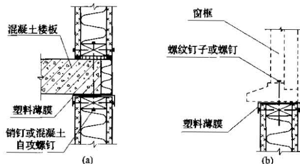
图 6.2.8 外墙体防渗、防潮构造示意图
