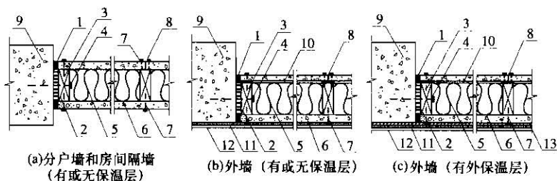
图 3.1.2 木骨架组合墙体构成示意图
