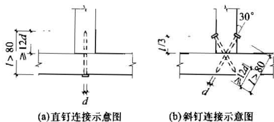
图 5.3.5 房间隔墙木骨架构件之间连接示意图
