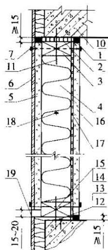
图 6 外墙竖向剖面图
