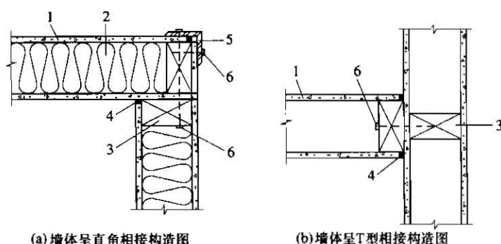
图 5.3.11 墙体相接构造示意图
