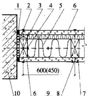
图 3 隔声内墙水平剖面图
