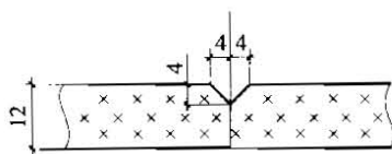
图 7 纸面石膏板的倒角
