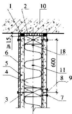
图 5 外墙水平剖面图
